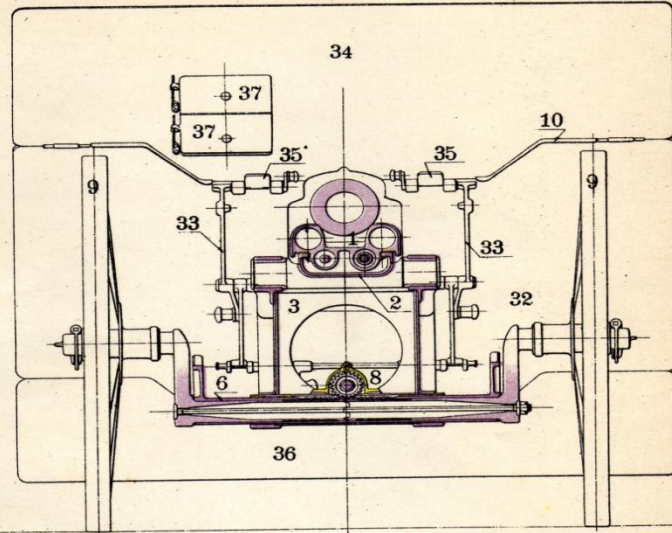
Coupe transversale.
